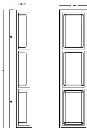
44650-018线条图
