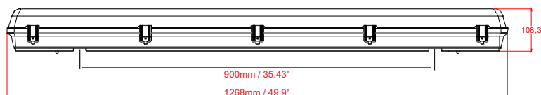
VTB2-4-557D Dimensions mm | 1268(L) x 167(W) x 108(D) inch | 49.9(L) x 6.6(W) x 4.3(D)
