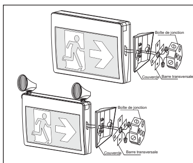
Support de côté Fig #6
