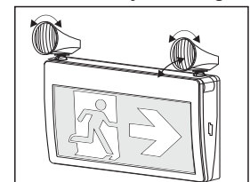
Montage mural avec la plaque arrière (Fig. 10)
