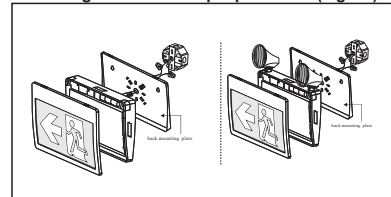
Montage mural avec la plaque arrière (Fig. 10)
